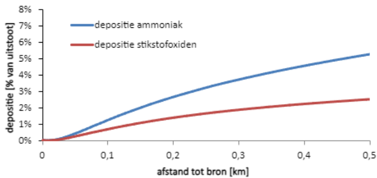
Figuur 2 Percentage van de totale stikstofuitstoot van een bron dat binnen 0,5 km neerkomt
