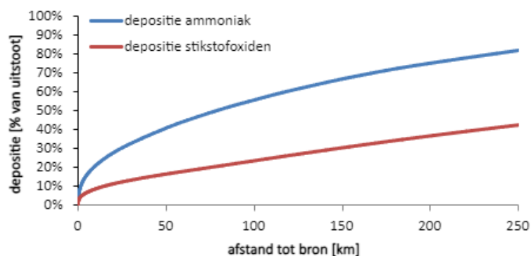
Figuur 3 Percentage van de totale stikstofuitstoot van een bron dat binnen 250 km neerkomt
