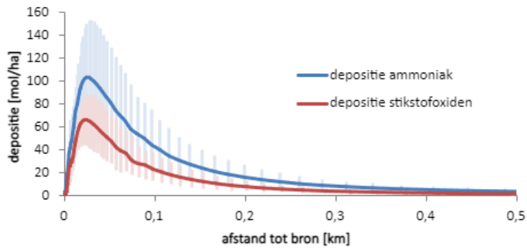
Figuur 1 Depositie van ammoniak en stikstofoxiden tot 0,5 km van de bron
